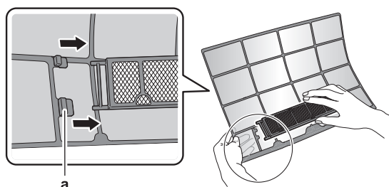
а Зажим
